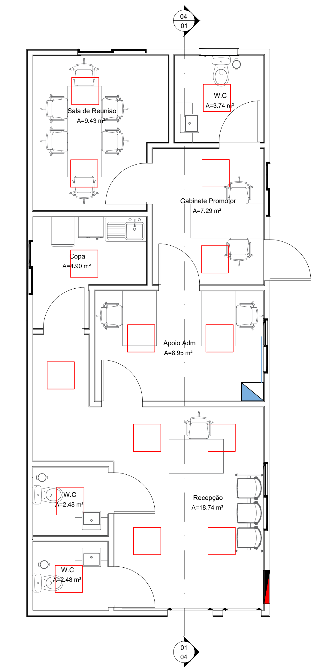
ILUMINAÇÃO esc. 1:50
