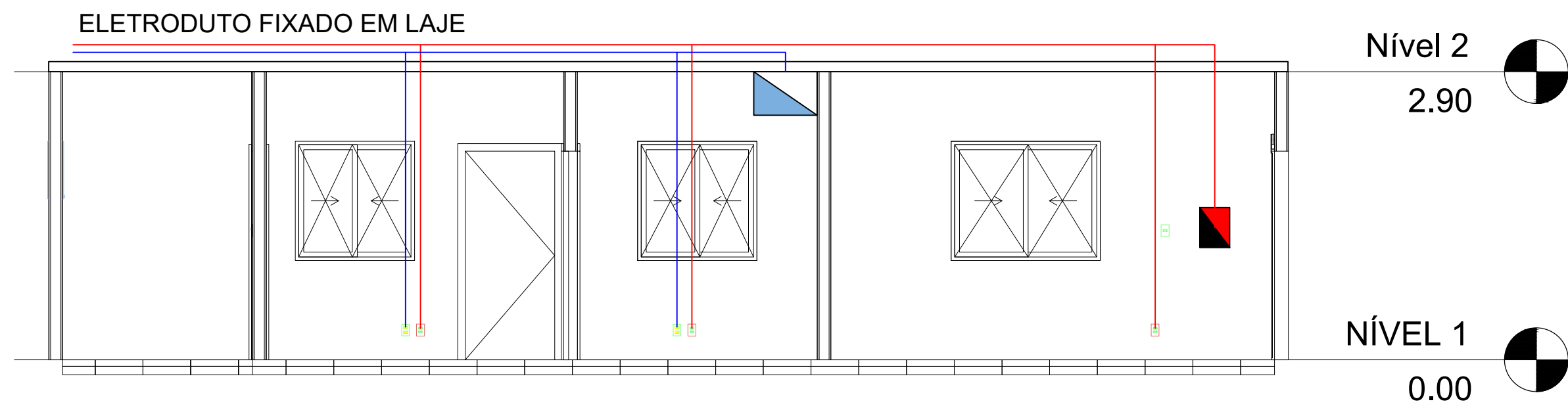
CORTE - 01 esc 1:50
