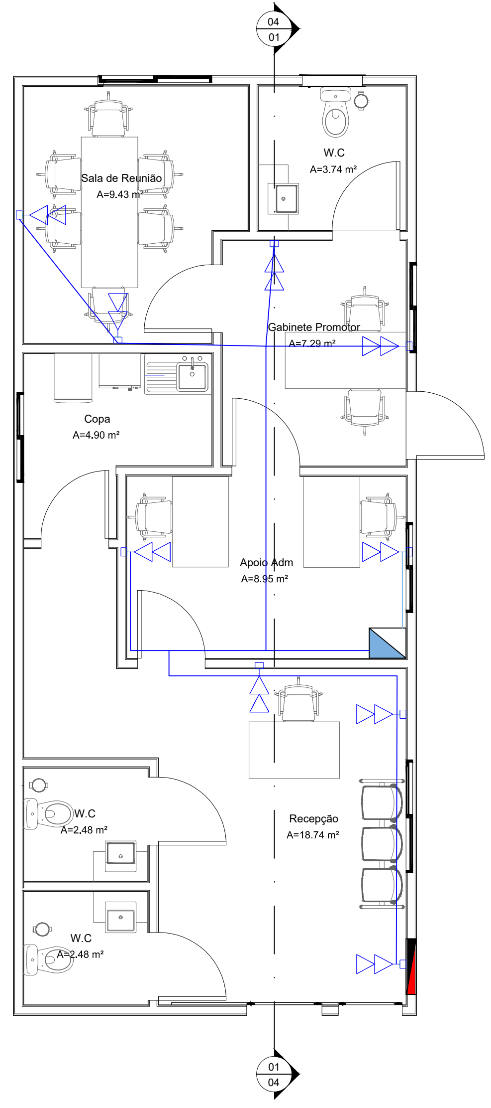
PONTOS DE LÓGICA esc 1:50
