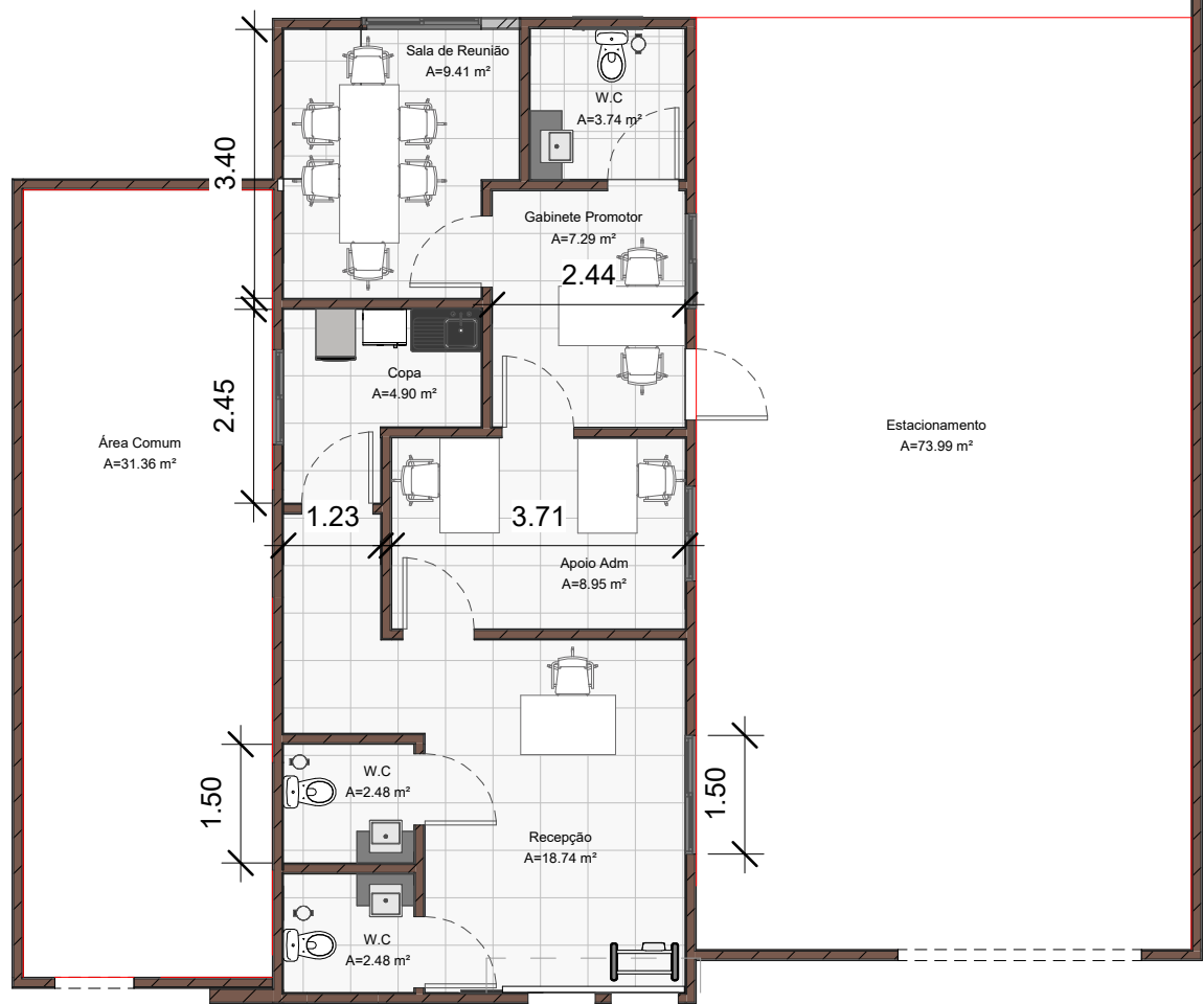
2 PLANTA BAIXA - NOVO 1 : 100
