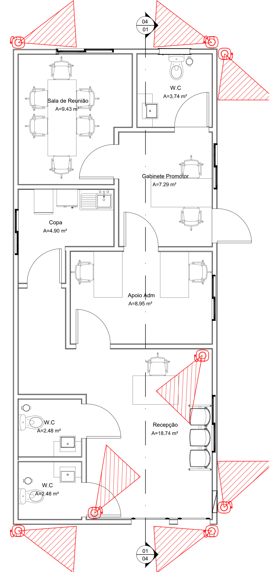
CÂMERAS DE SEGURANÇA esc 1:50
