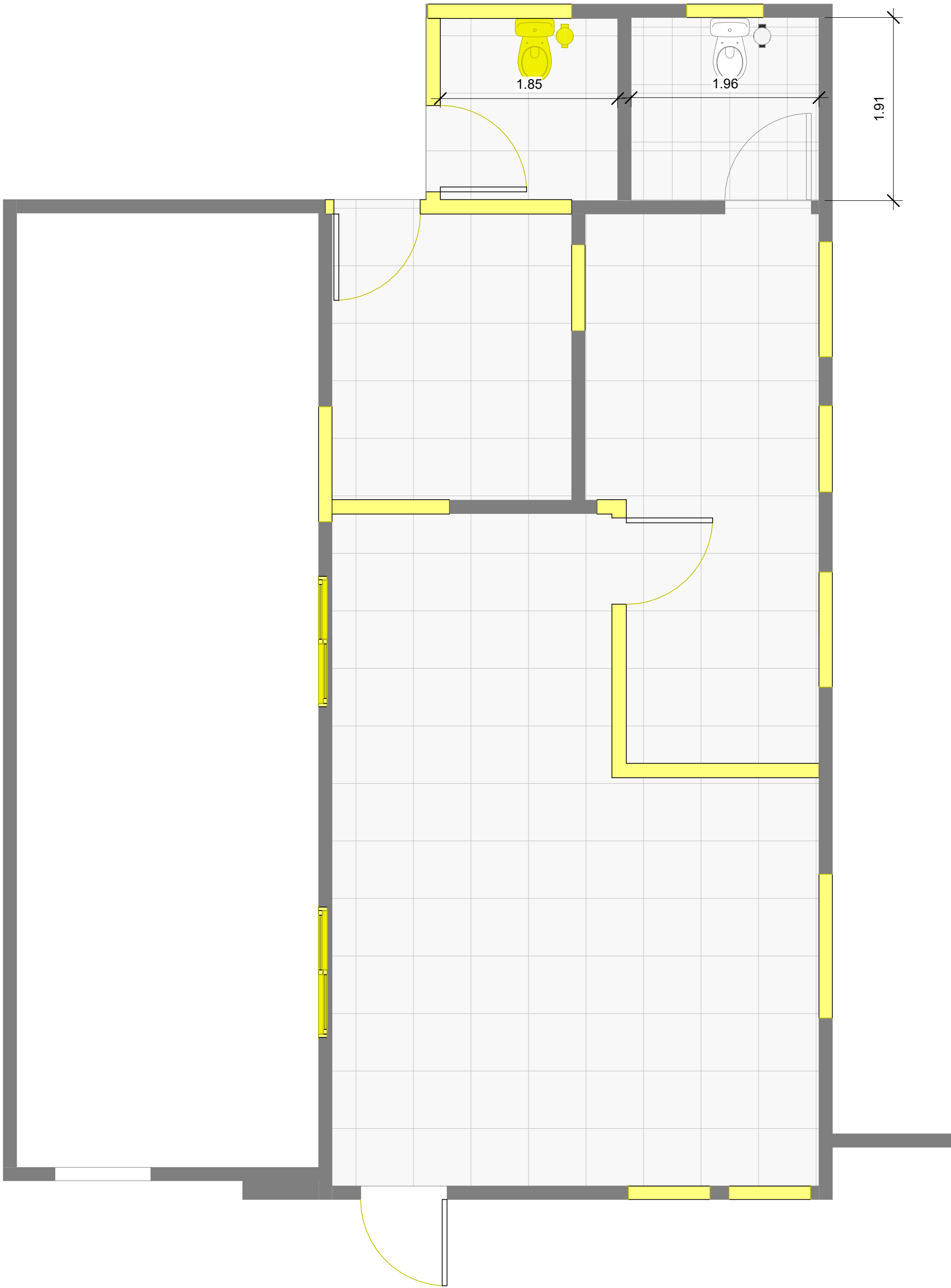
1 DEMOLIR 1 : 40
