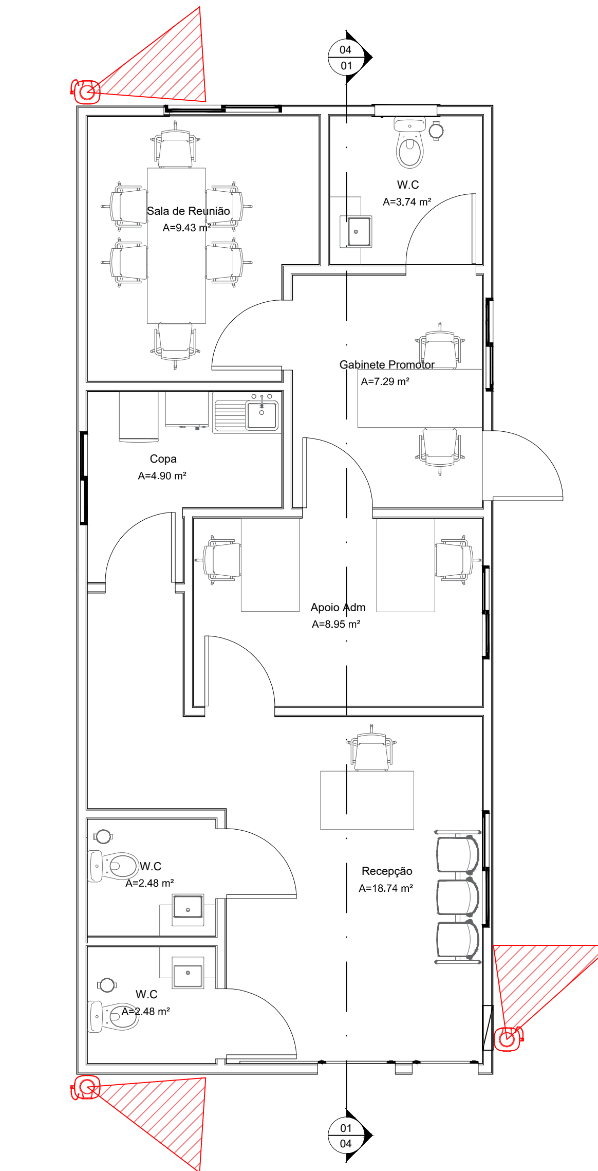
REFLETORES esc. 1:50
