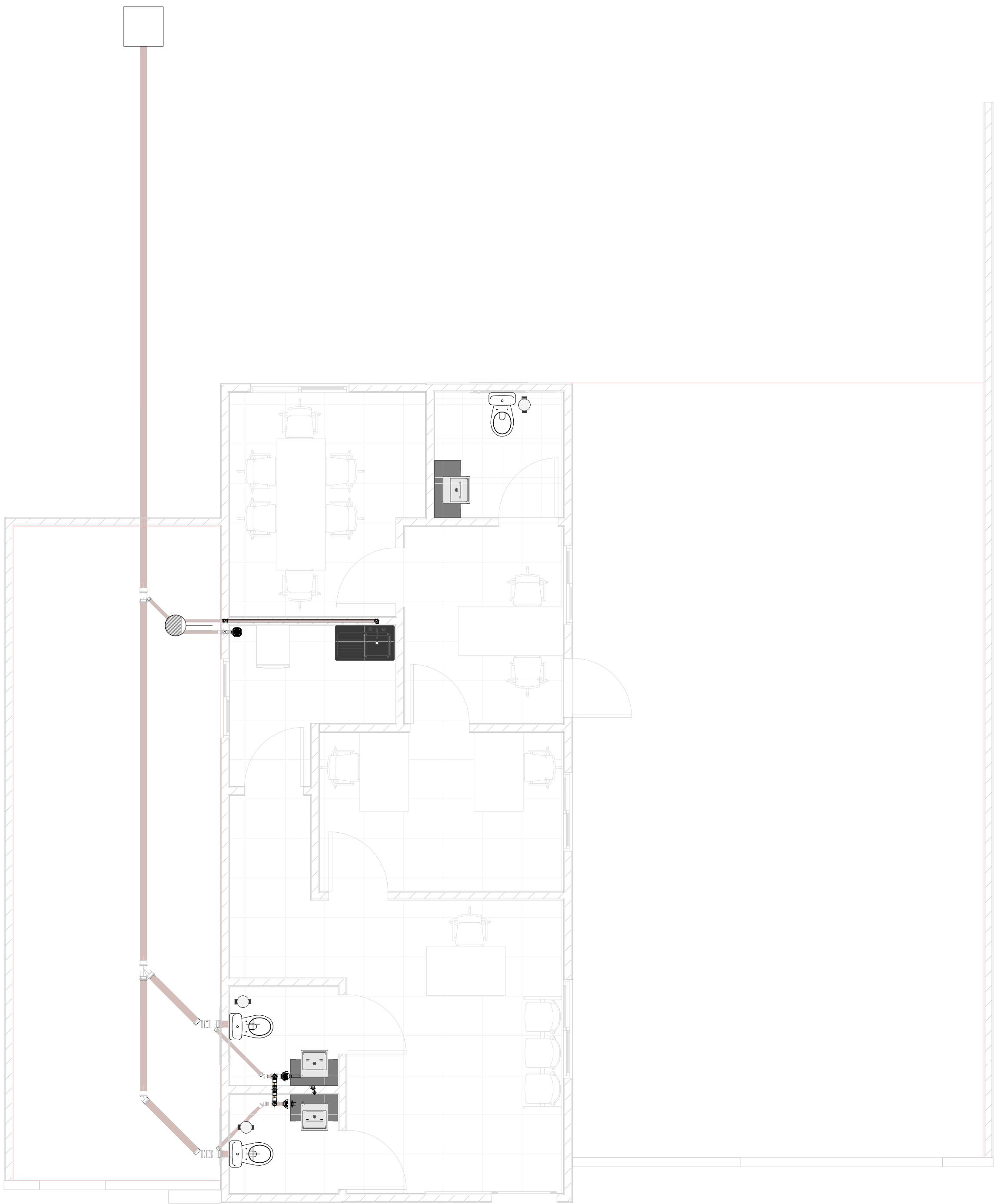
1 ESGOTO - NOVO 1 : 50
