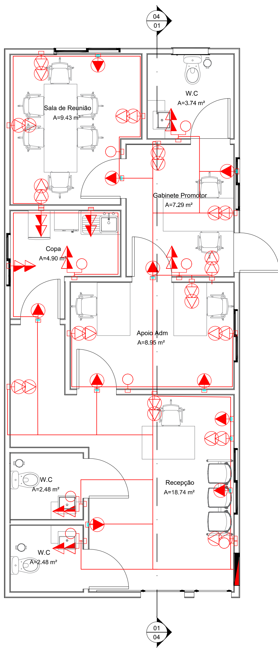
PONTOS DE ELÉTRICA esc 1:50
